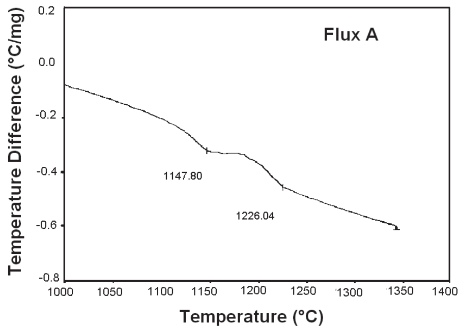
Fig. 5. DTA diagram of flux A.
