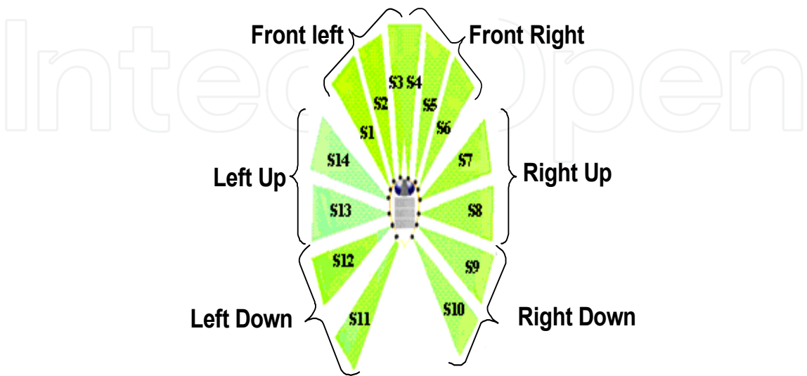
Fig. 21. IR sensors arrangement.
