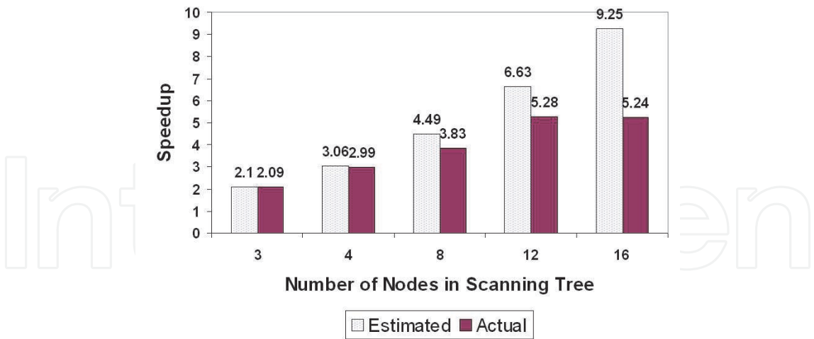
Fig. 6. Estimated vs. Actual Speedup Values.
