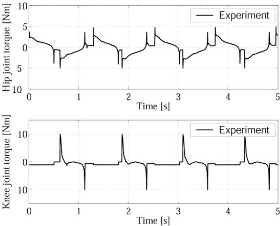
Fig.19. Joint input torque (Hase T. & Huang, Q., 2005).
