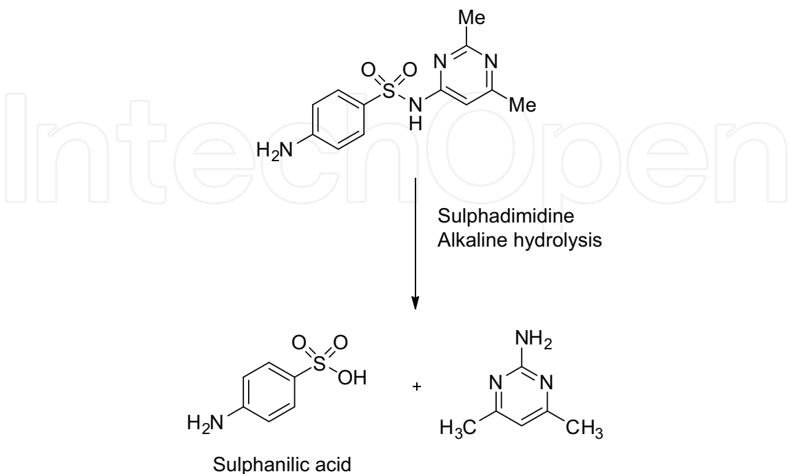
Fig. 11. Titrimetric analysis of Sulphadimidine
