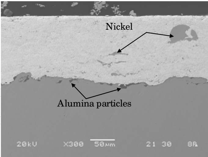
Fig. 2. WCCoCr + SP+ G coating
