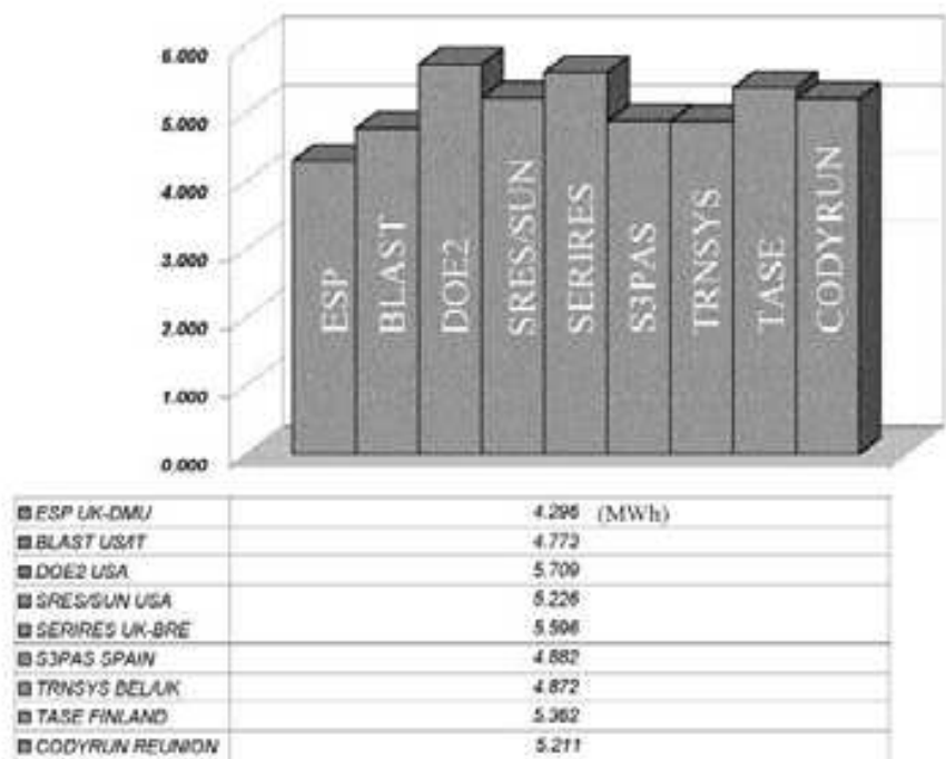
Fig. 5. Exemple of BESTEST result
