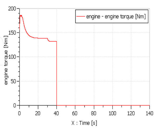
(d) Variation of torque at the heat engine shaft
