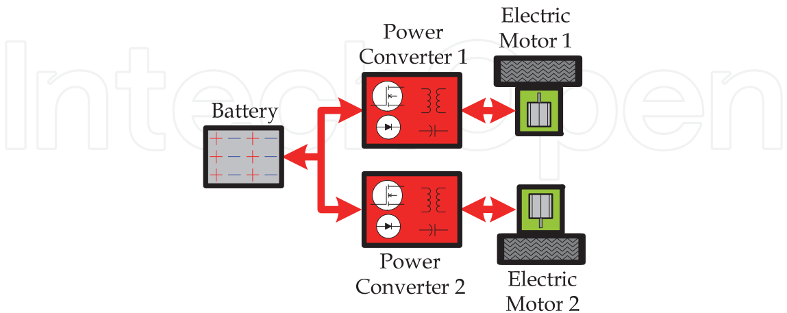
Fig. 7. Two-motor BEV
