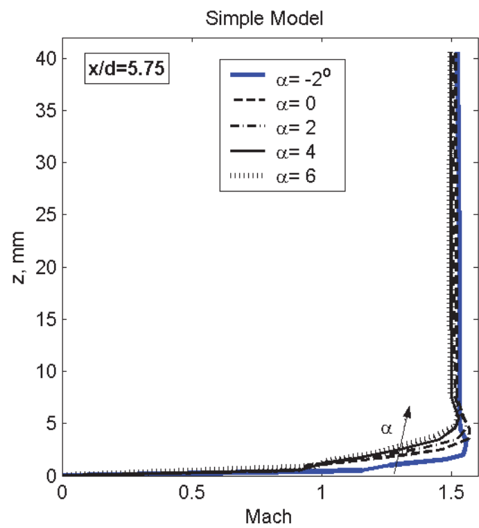
a) x/d=5.75
