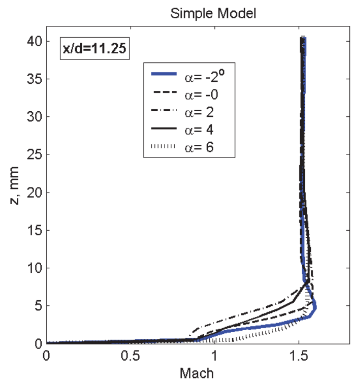
b) x/d=11.25
