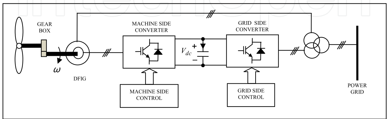
Fig. 13. DFIG WECS
