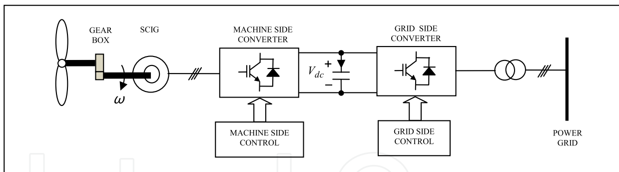
Fig. 10. SCIG WECS
