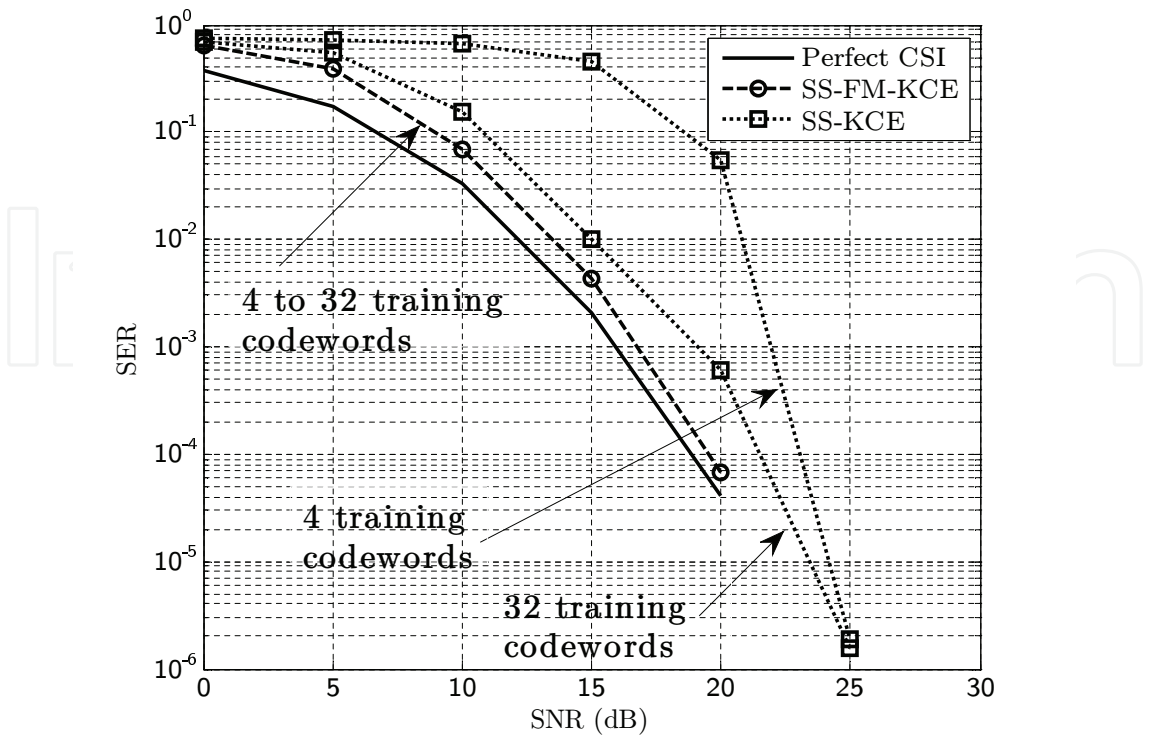
Fig. 10. Symbol error rate for SS-KCE and FM-KCE.
