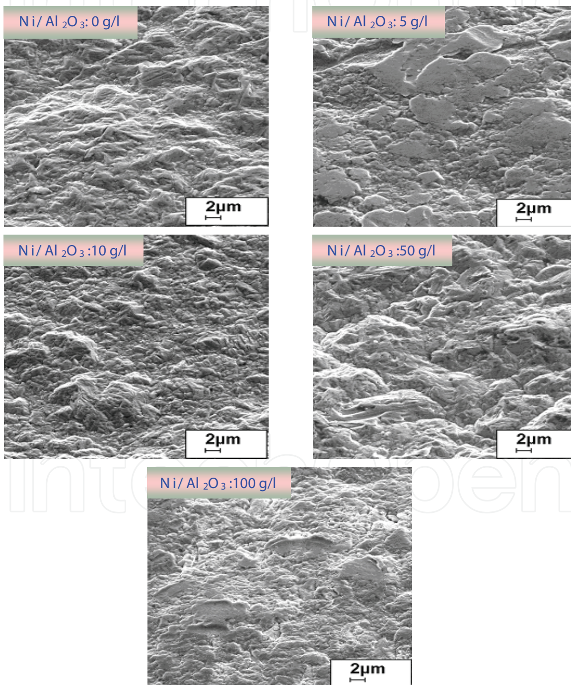
Fig. 2. SEM images of Ni/ Al 2 O 3
