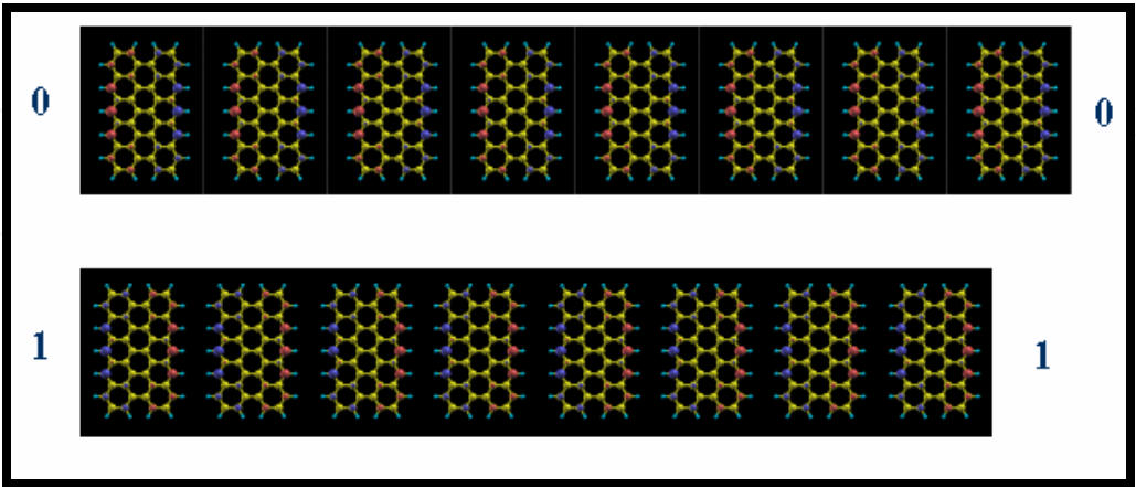
Fig. 14. Molecular wire.
