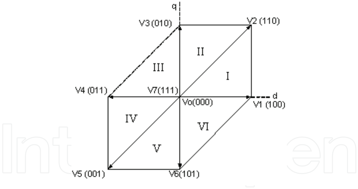
Fig. 5. Space-vectors hexagon.
