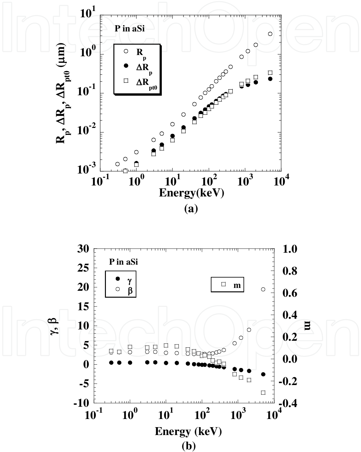
Fig. 18. Moment parameters of P ion implantation profiles.
