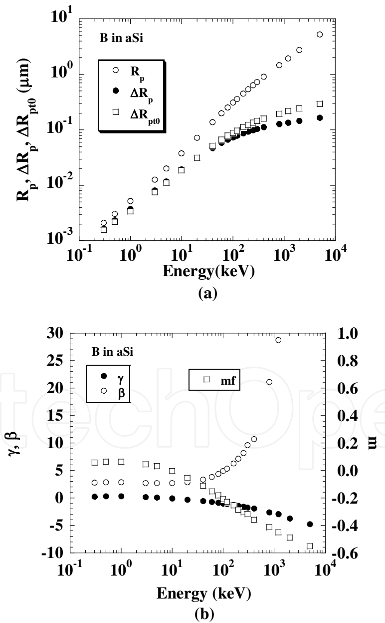
Fig. 17. Moment parameters of B ion implantation profiles.
