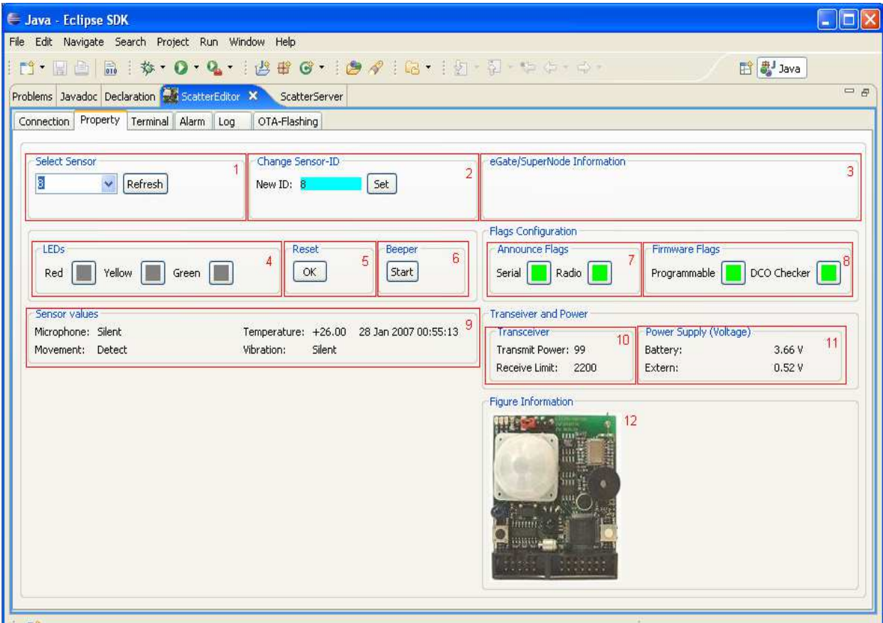
Fig. 16. Property Tabfolder
