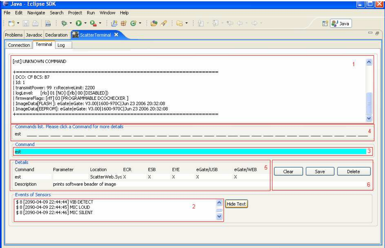
Fig. 17. Terminal Tabfolder
