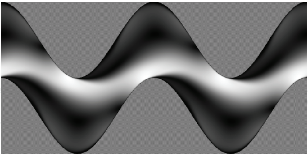
(a) |\vec{v}|
