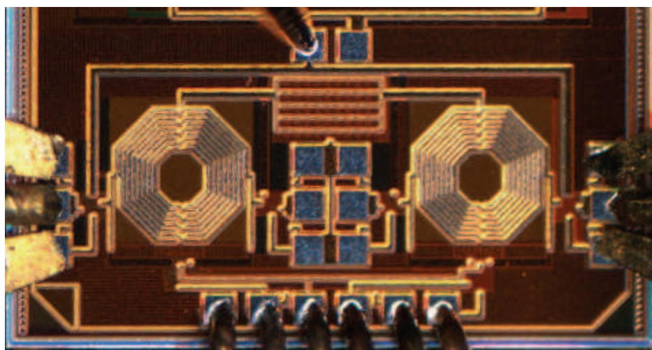
(b) CR-QVCO die photo.
