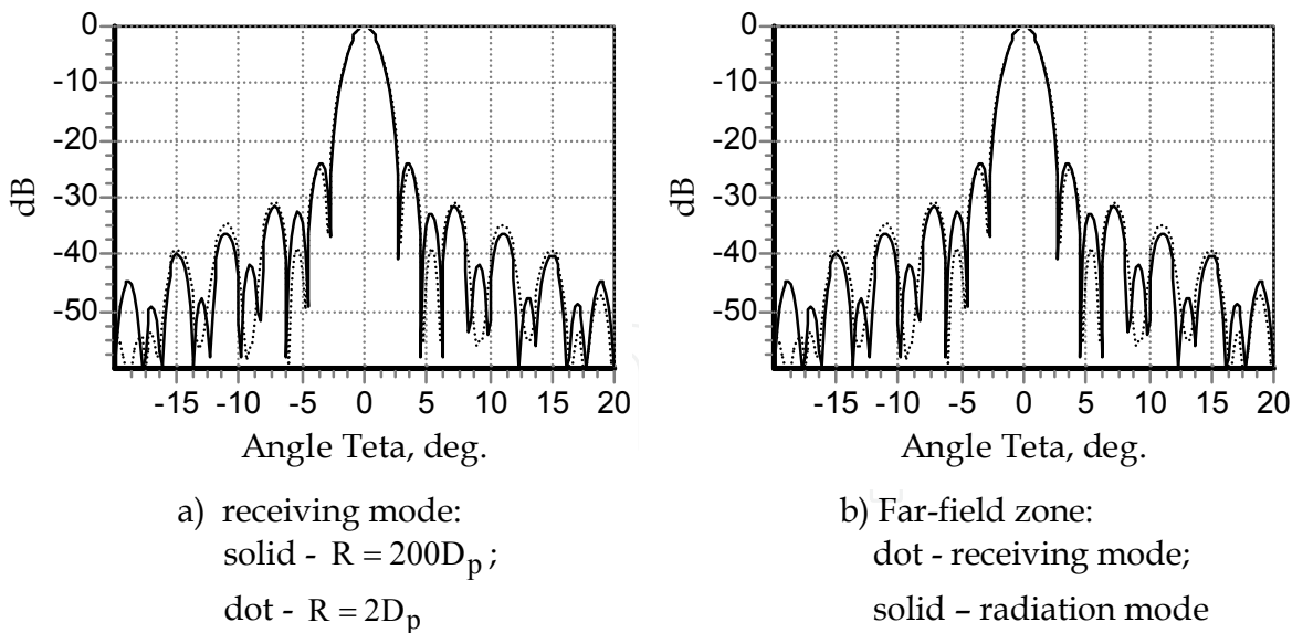
Fig. 12. Antenna diagrams
