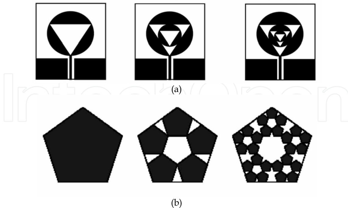
Fig. 19. The fractal UWB antennas
