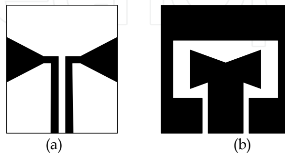
Fig. 10. The UWB bowtie antennas
