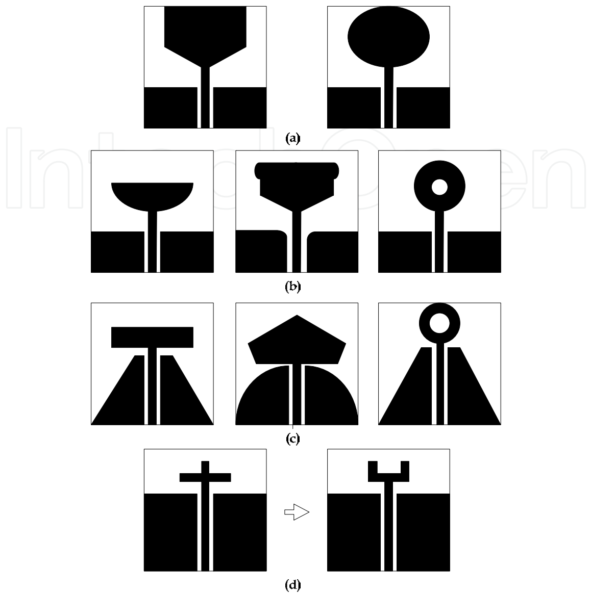
Fig. 14. The CPW-fed monopole UWB antennas
