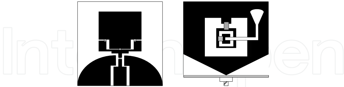
Fig. 29. Active UWB antennas
